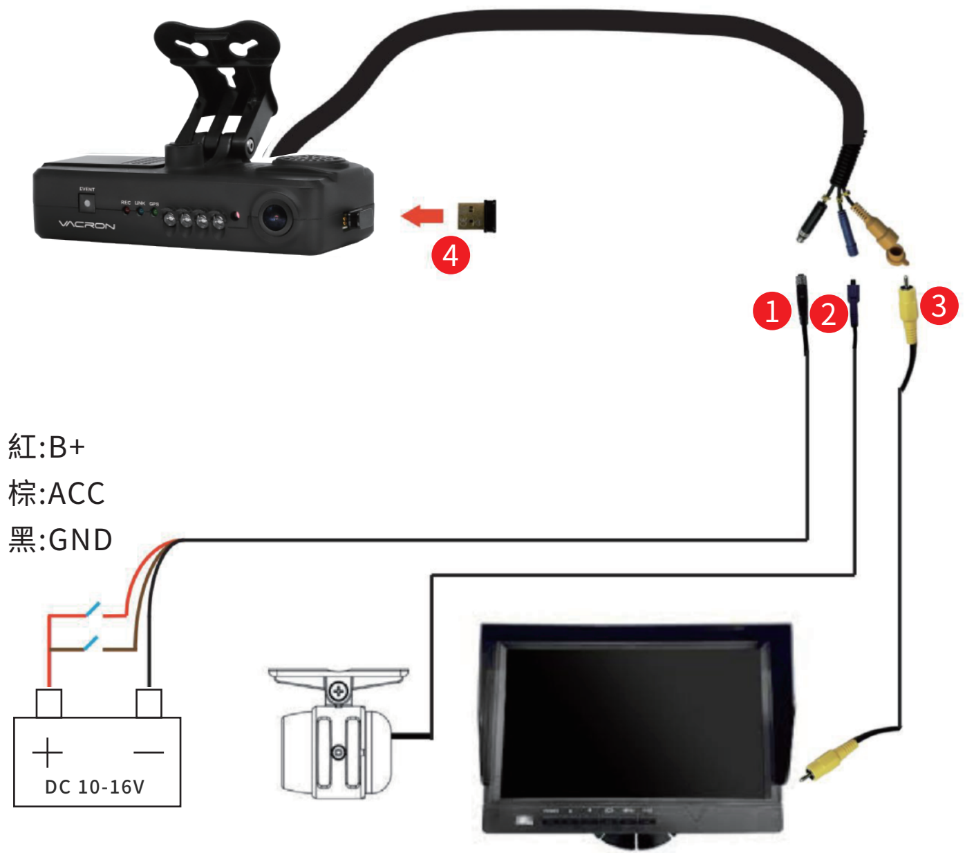
配線示意圖
