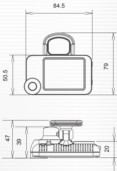
■外觀尺寸圖 單位:mm
