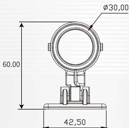
外觀尺寸圖 單位：mm
